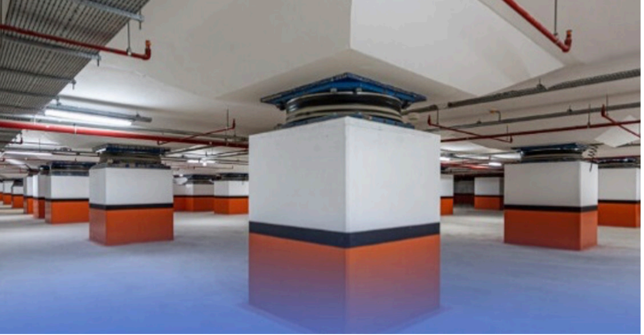
Sismik izolatör uygulaması [13]
